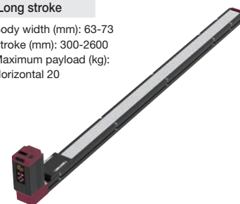
EC-DB
